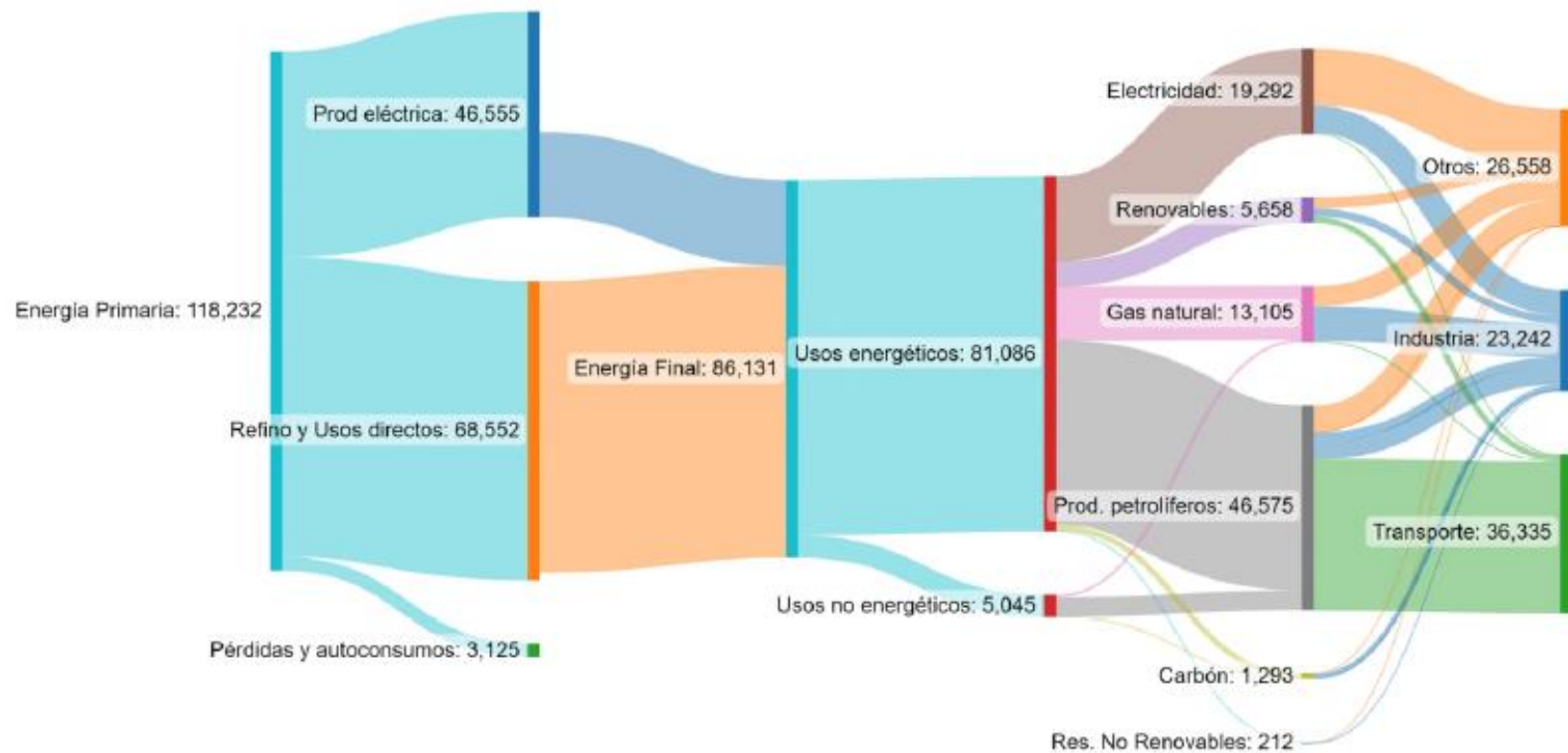
Figura 1.2. Diagrama Sankey de la energía en España en 2022. Cifras en kteq.
