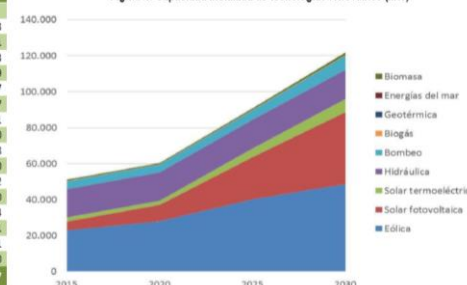
Figura 4: Capacidad instalada de tecnologías renovables (MW)
